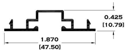
9085 TAPA BOLSA
