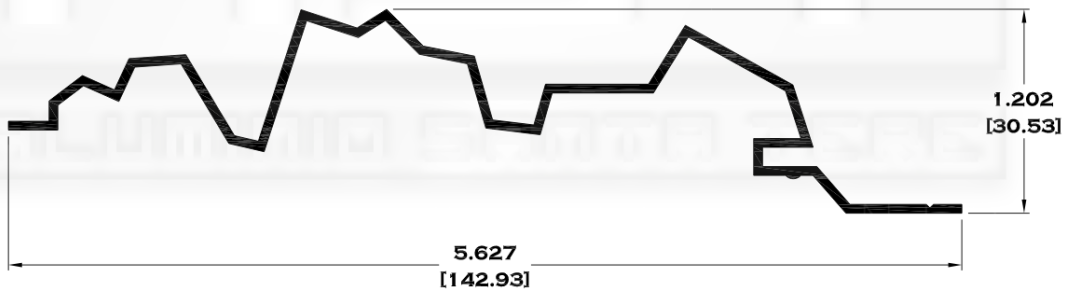
8380 DUELA GRAFICADA
