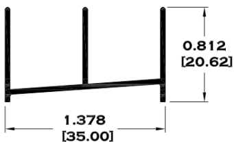
11387 RIEL
