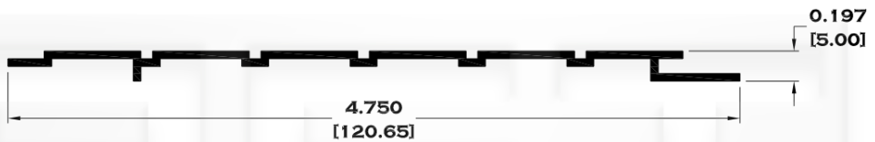
6775 DUELA ENTRECALE
