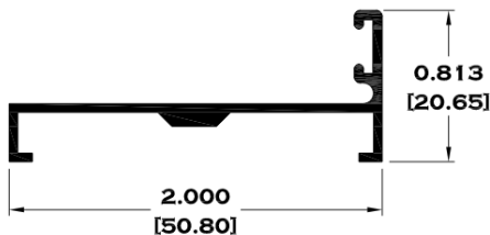
5844 BATIENTE
