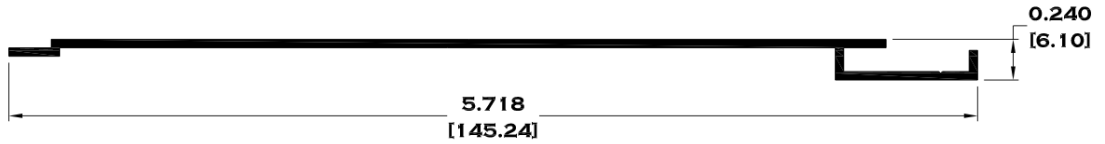
6617 DUELA LISA
