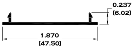
4051 TAPA LISA
