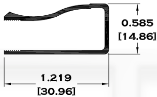
9525 MARCO ECONOMICO
