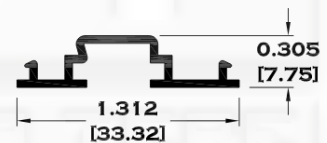
9075 TAPA BOLSA
