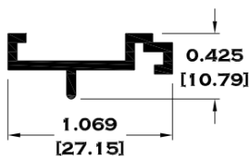
9966 ADAPTADOR MOSQUITERO
